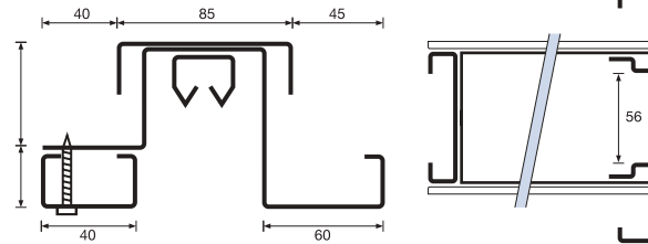
SECCIÓN PERFIL Y RIEL
