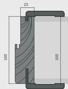
Mínima apertura contramarco
