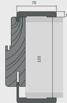
Máxima apertura contramarco
